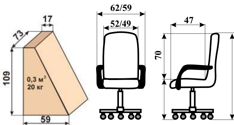
Размеры кресла Сенатор/Надир
