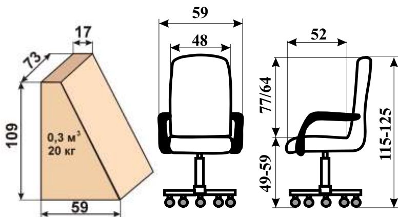
Размеры кресла стандартной высоты/с низкой спинкой
