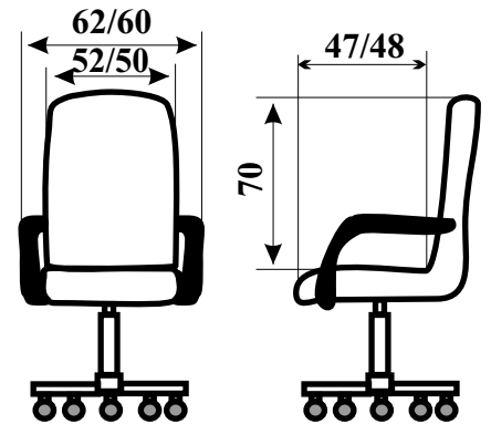
Размеры кресла Тунис/Зодиак
