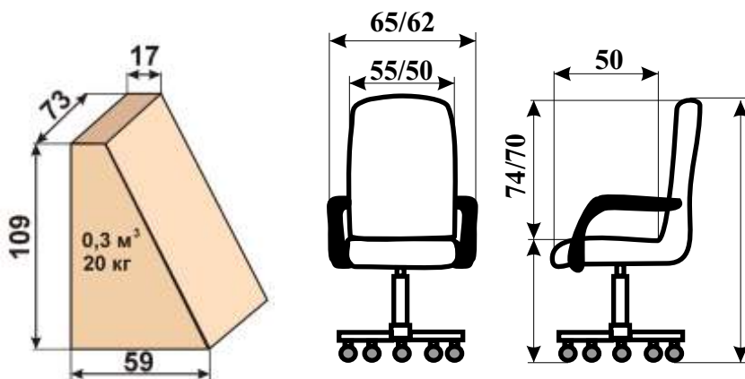
Размеры кресла Мерседес/Рим
